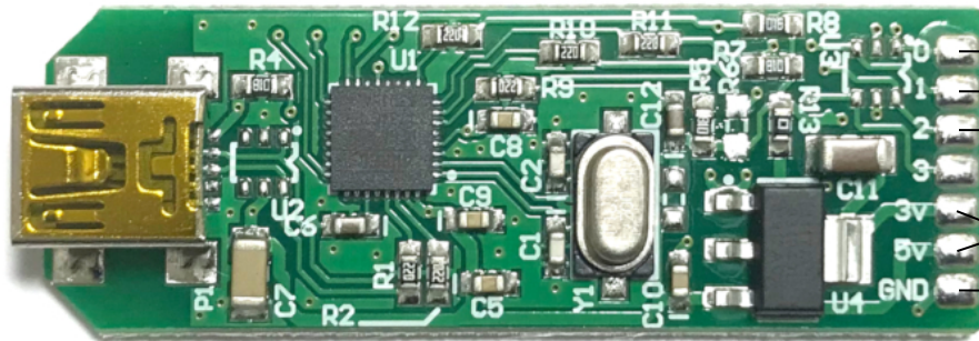
BRD-VBOY-USB_v2
