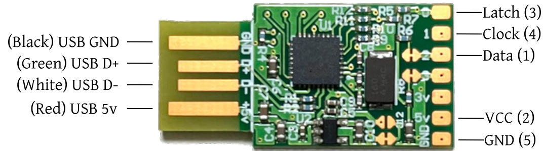
BRD-VBOY-USB_v2-SLD
